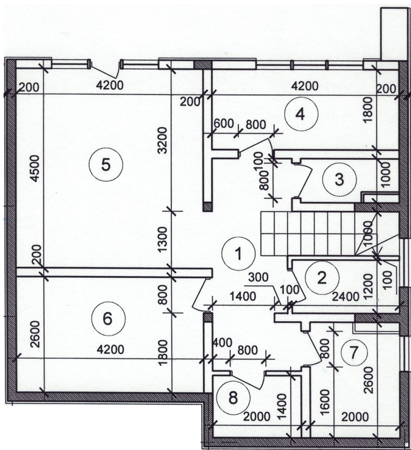
План цокольного этажа
